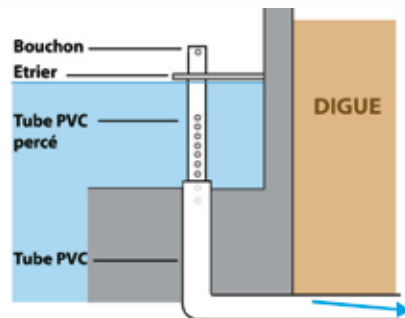
(e) Le débit réservé : schéma du système de régulation
